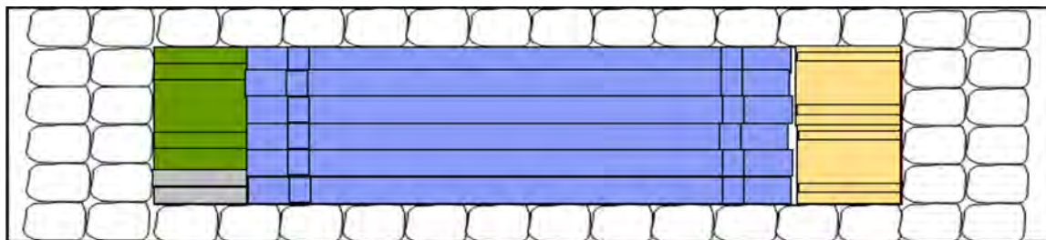
Схема расположения груза на борту Франкоп .
