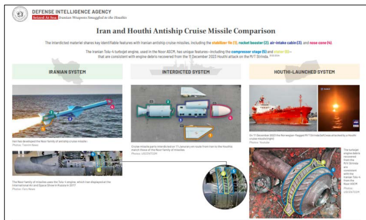
השוואת רכיבים של טילי שיוט נגד ספינות חות'ים ואיראניים (סוכנות המודיעין של משרד ההגנה האמריקאי, 10 ביולי 2024)
